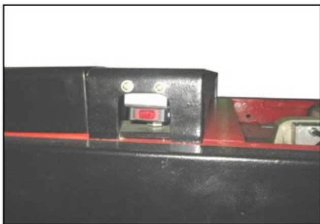
Figura 26 (posição fotocélula)
